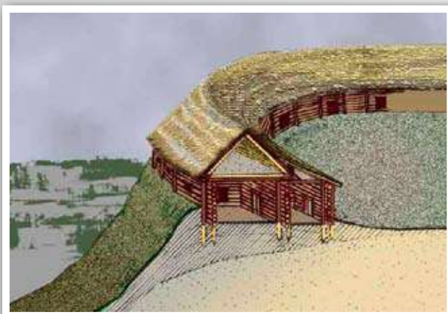
Pav. 2. Aukštadvario piliakalnio gynybinės sienos rekonstrukcija.
